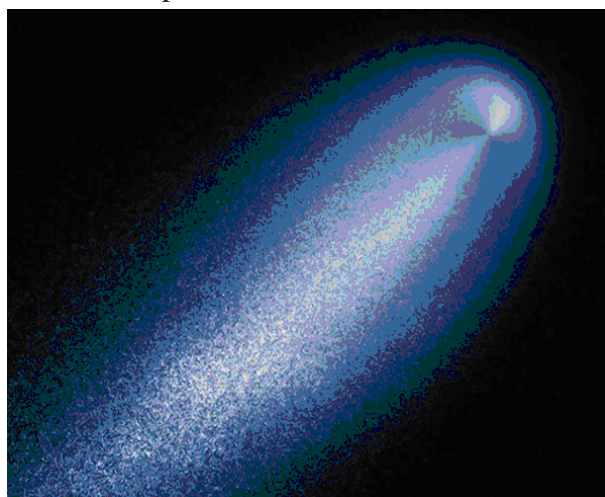
1. La cometa ISON, fotografata a maggio 2013. (Per gentile concessione della NASA)
