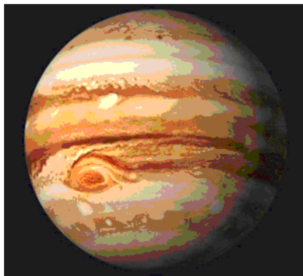
2. Giove, in basso a sinistra la Grande Macchia Rossa
